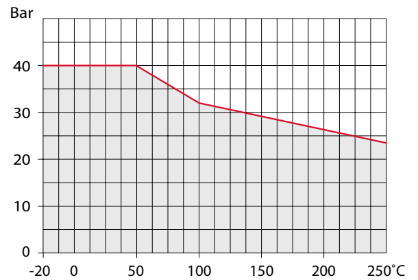
PN 40: Beidseitig Flansch – DN 15 - 50
