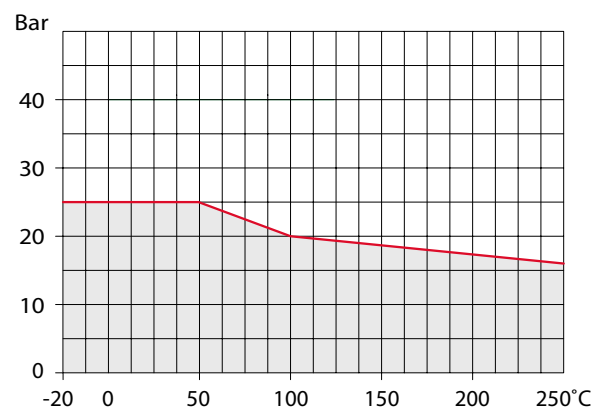
PN 25: Beidseitig Flansch – DN 65 - 200
