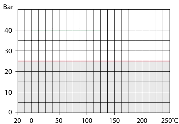
PN 25: Beidseitig Schweißende – DN 65 - 200
