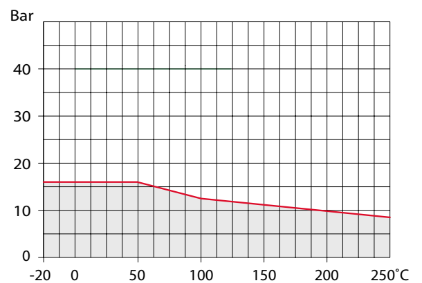
PN 16: Beidseitig Flansch – DN 65 - 200
