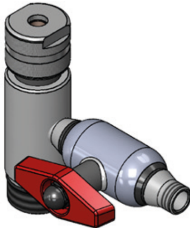
Aufbau der Abdichtung für die Bohrstangendurchführung:
