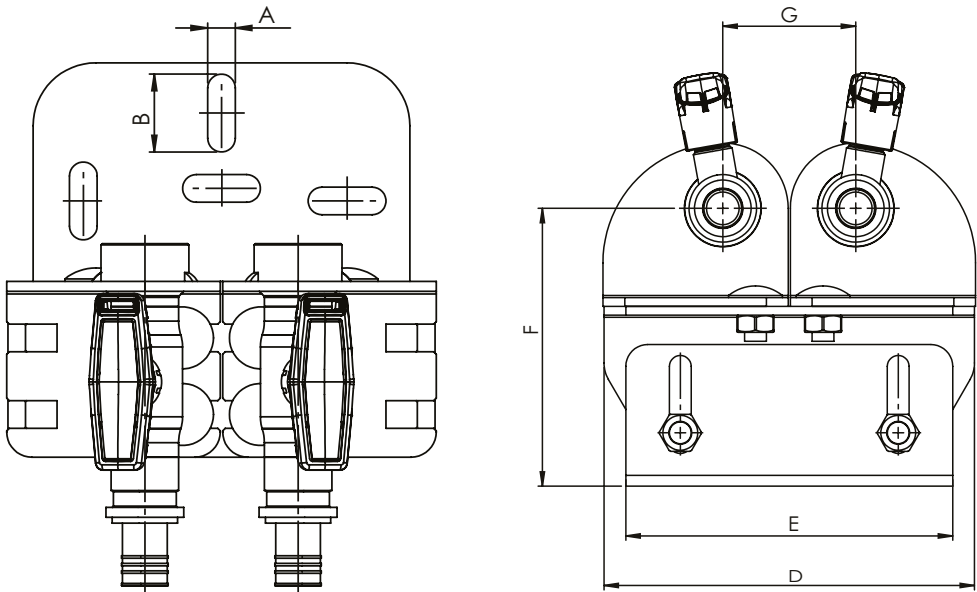
Abmessungen
