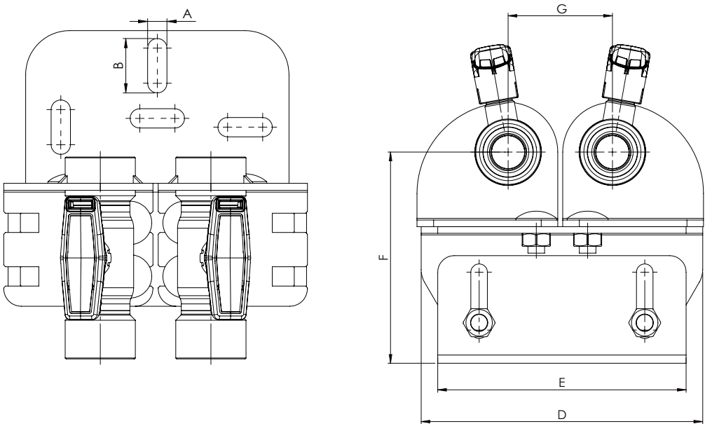
Abmessungen
